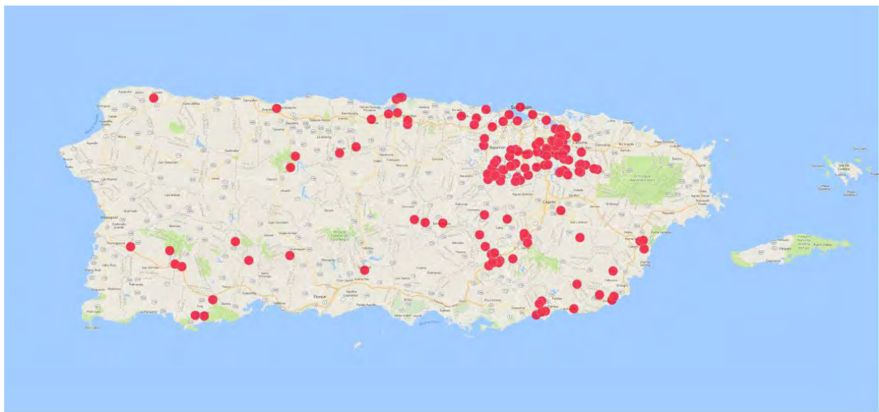
Figura 69. Instalaciones de la AAA con daño en generador a causa de los Huracanes Irma y María 170
