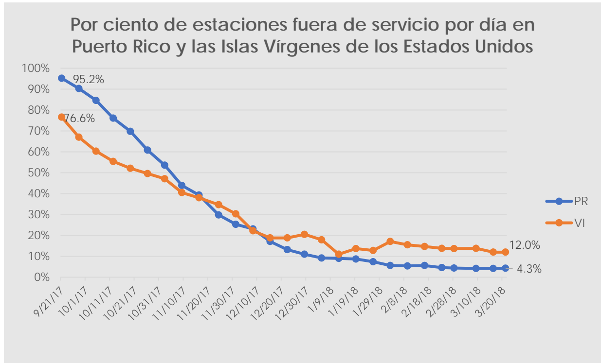
Figura 58. Fuente: Impacto en las comunicaciones de las tormentas de 2017 en el Atlántico
